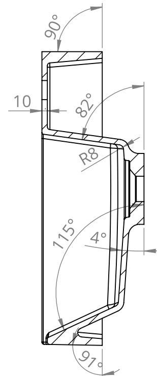
PRZEKRÓJ G-G SKALA 1 : 7
