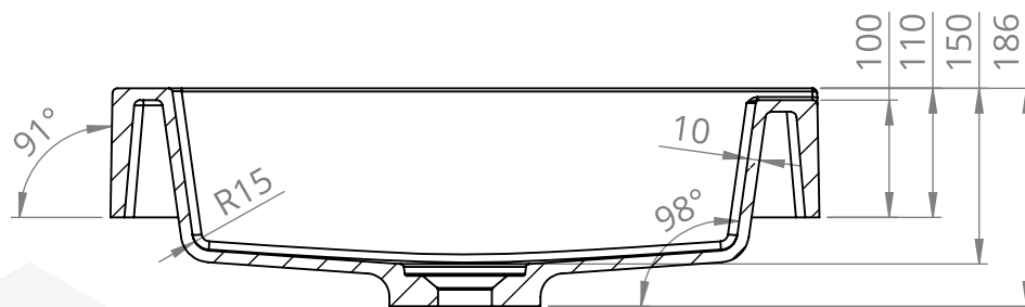
PRZEKRÓJ H-H SKALA 1 : 7
